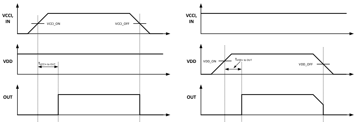
图 8-5. V_{CCI}/V_{DD} UVLO 上电延时
